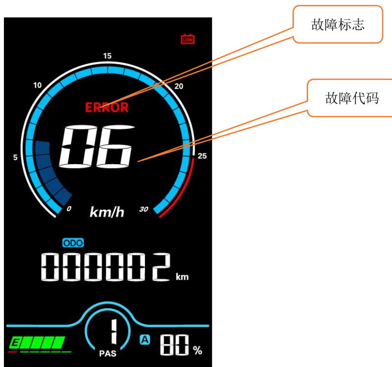
图示说明：故障：ERROR 标志，06 表示故障代码
