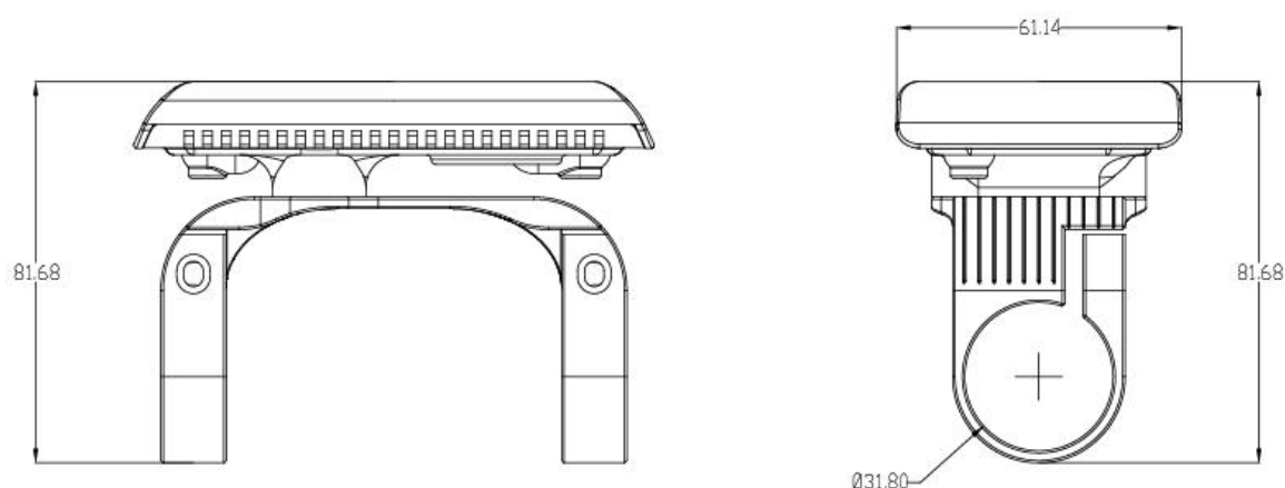
正视图
